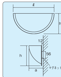
〈取付け図〉
