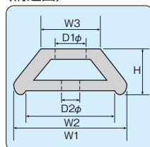
〈構造図〉
