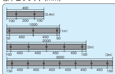
標準ピッチ穴 (mm)
