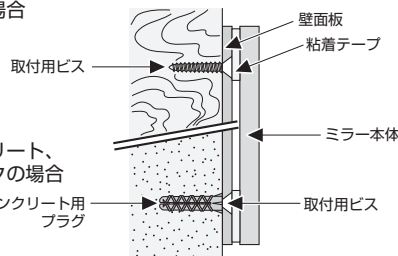
〈ビス等で取付ける場合〉
