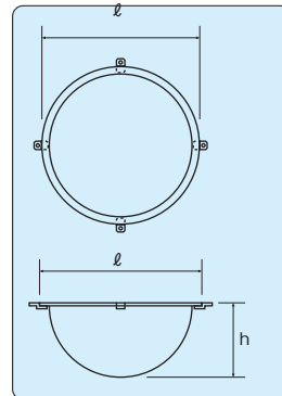
〈取付け図〉
