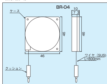
〈構造図〉
