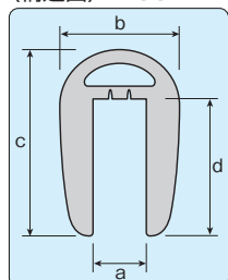
〈構造図〉 H-08~22
