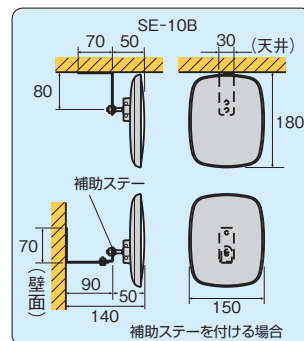
〈取付け図〉
