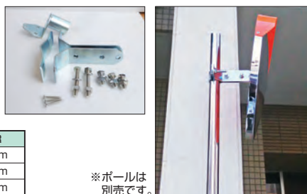
〈取付け例〉
